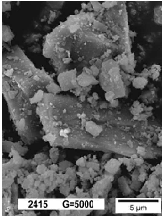
Fig. 1 - SEM of limestone-quarry fines (13).
